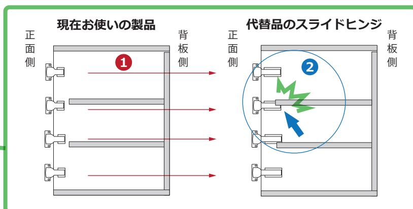
キャビネットを横から見た図
